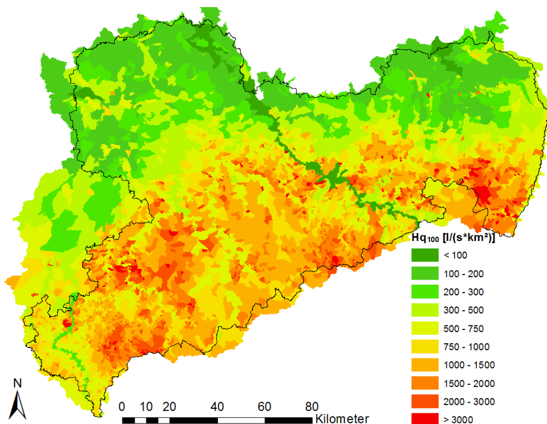
Abbildung 38: 100-jährliche Hochwasserscheiteldurchflusspenden Hq_{100} an den Zufluss- (oben) und Ausflussknoten (unten) der Teileinzugsgebiete
