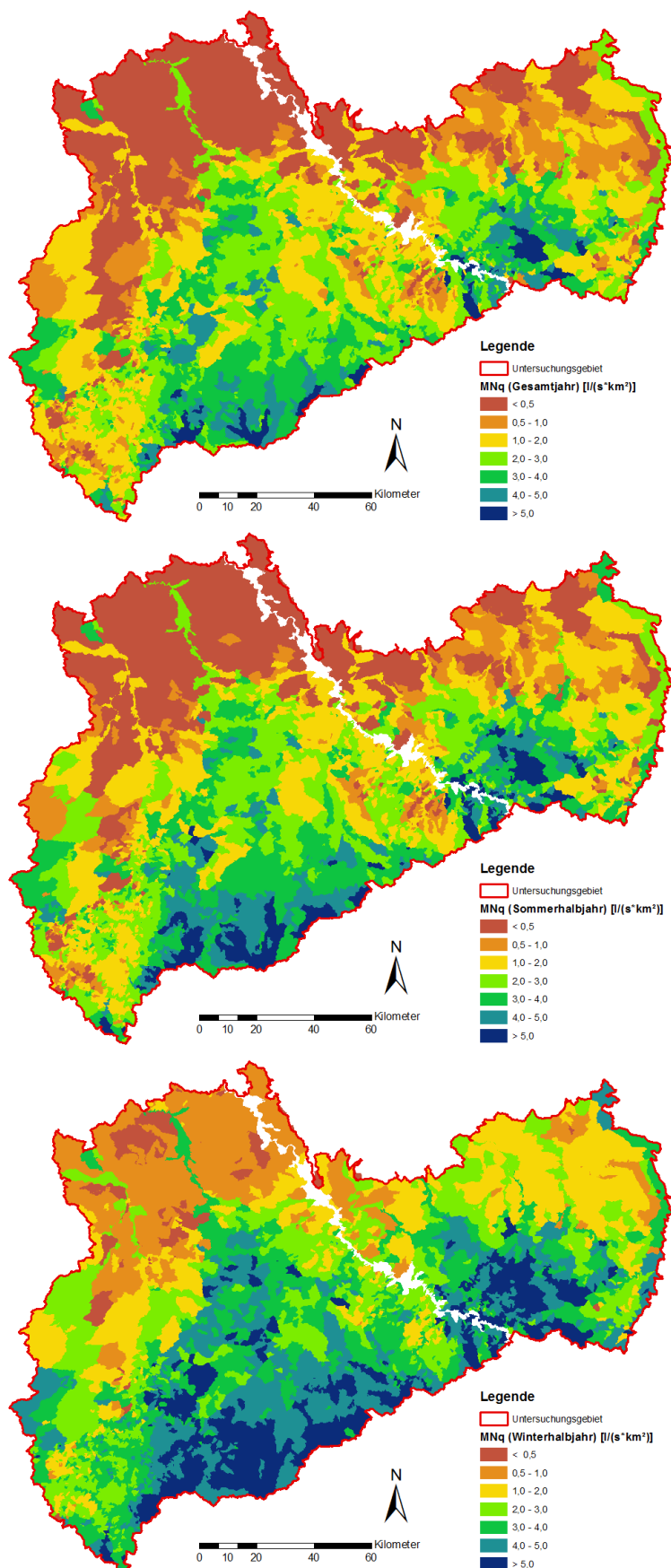
Abbildung 25: Vollständig plausibilisierte Durchflussspenden MNq der Teileinzugsgebiete der Ausflussknoten für das Gesamtjahr (oben), das Sommerhalbjahr (Mitte) und das Winterhalbjahr (unten)
