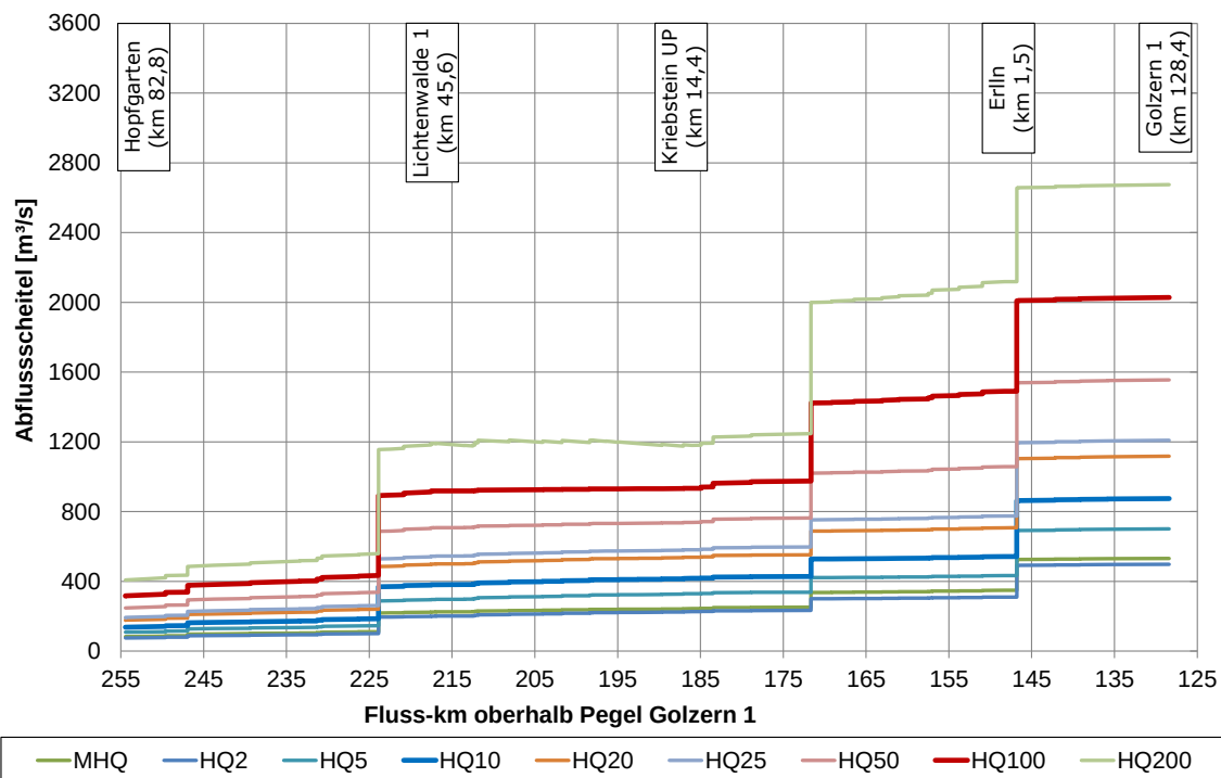
Abbildung 33: MHQ- und HQ 2 - bis HQ 200 -Längsschnitte der Zschopau, Freiberger und Vereinigte Mulde vom Pegel Hopfgarten bis zum Pegel Golzern 1
