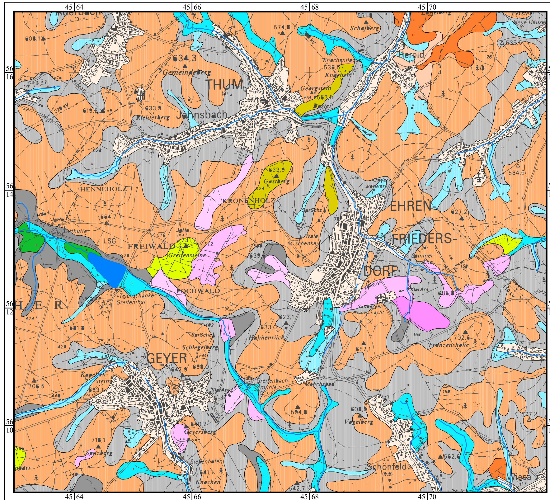
Abb. 6: Vereinfachte Bodenkarte
