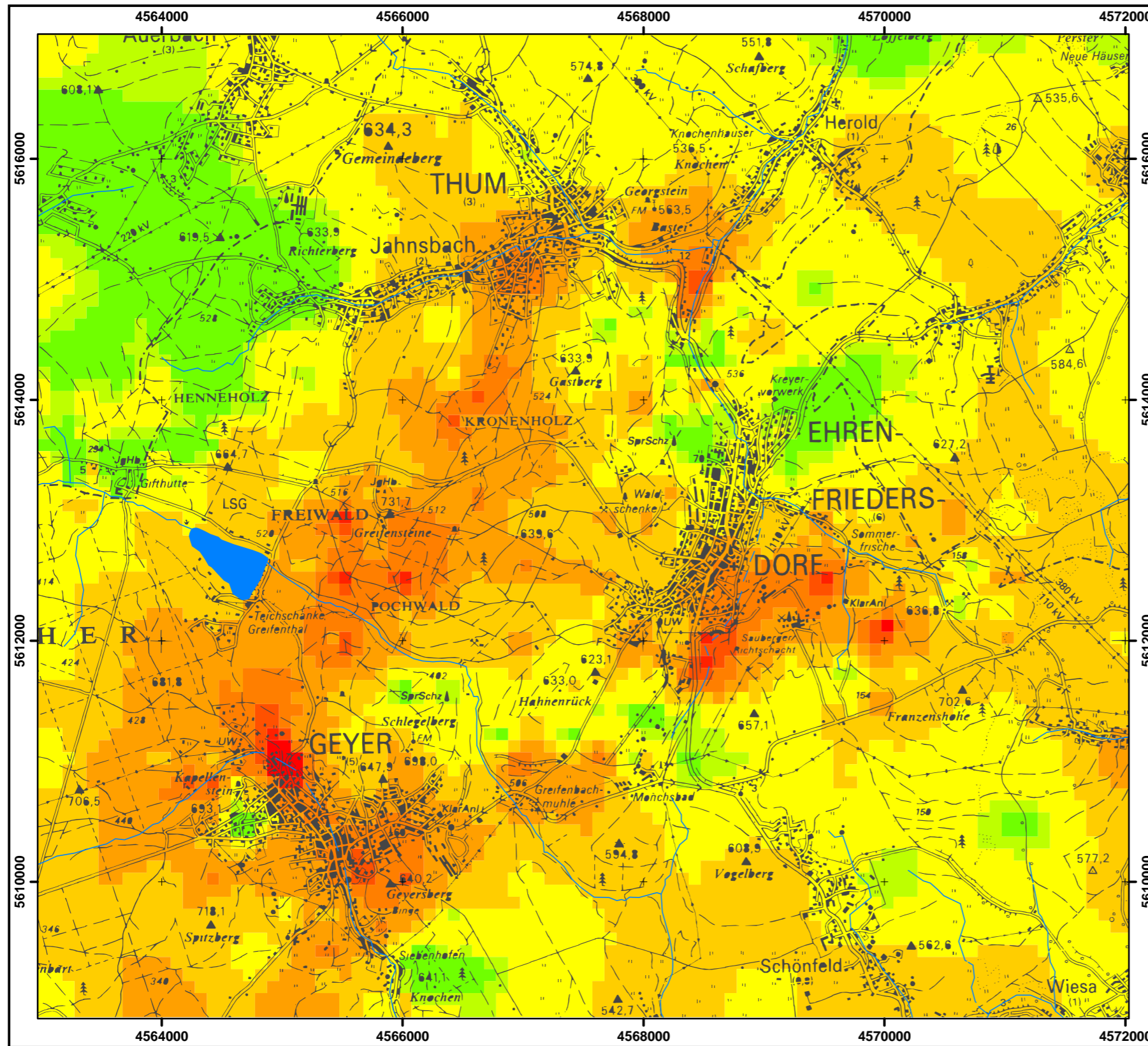
Abb. 40: Thallium im mineralischen Oberboden
