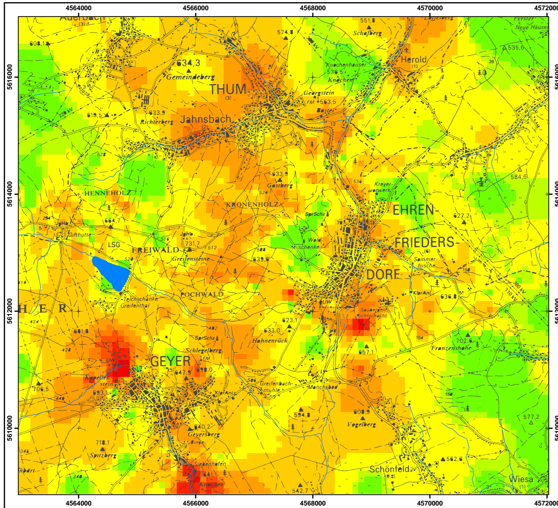
Abb. 35: Blei im Unterboden
