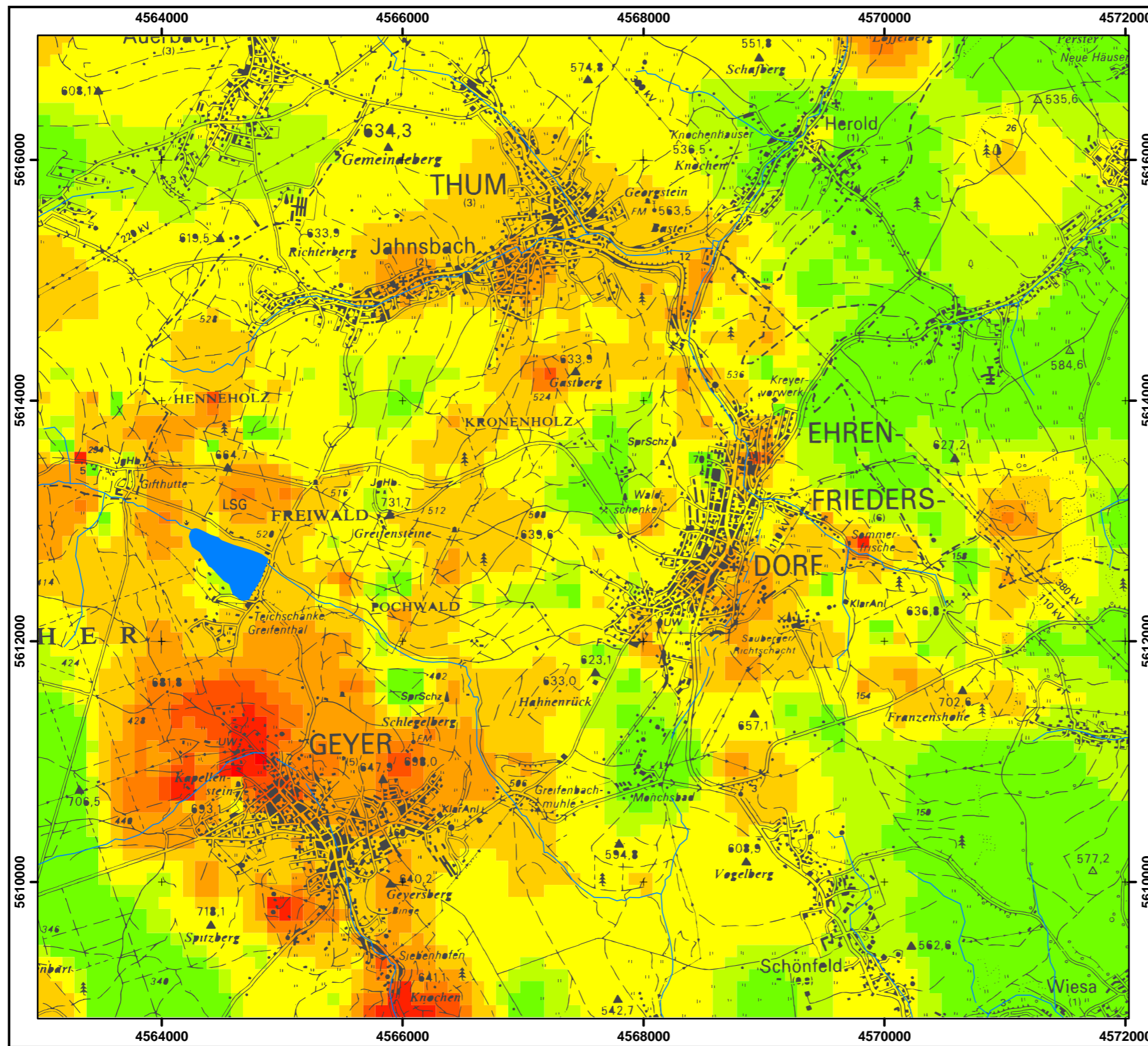
Abb.30: Blei im mineralischen Oberboden
