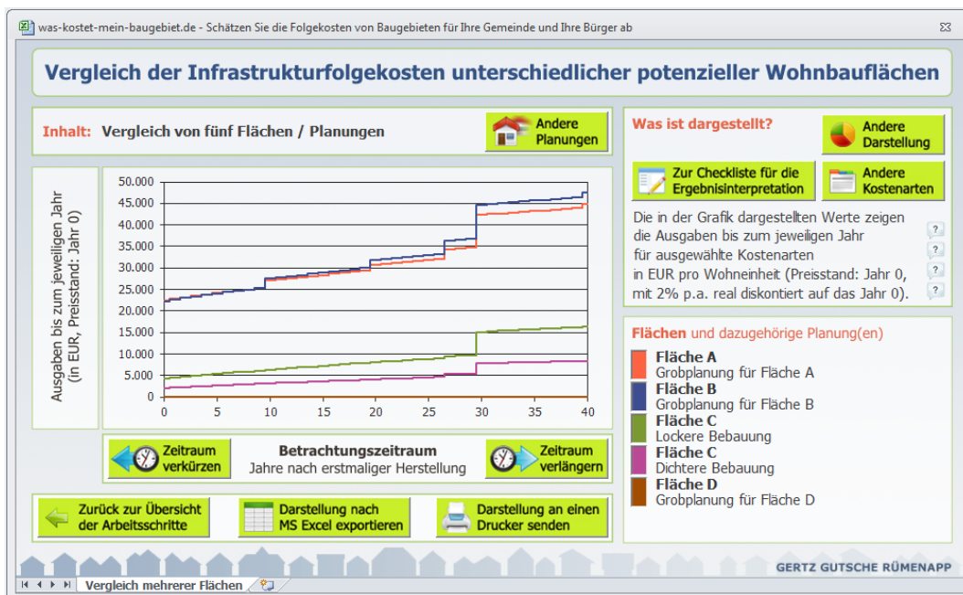
Abbildung 47 Vergleich des Kostenanteils der Gemeinde pro Wohneinheit
