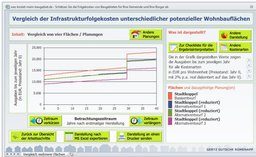
Abbildung 37 Vergleich der vier Entwürfe: Kosten der Gemeinde pro Wohneinheit
