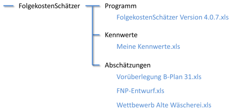
Abbildung 1 Vorgeschlagnene Ordnerstruktur
