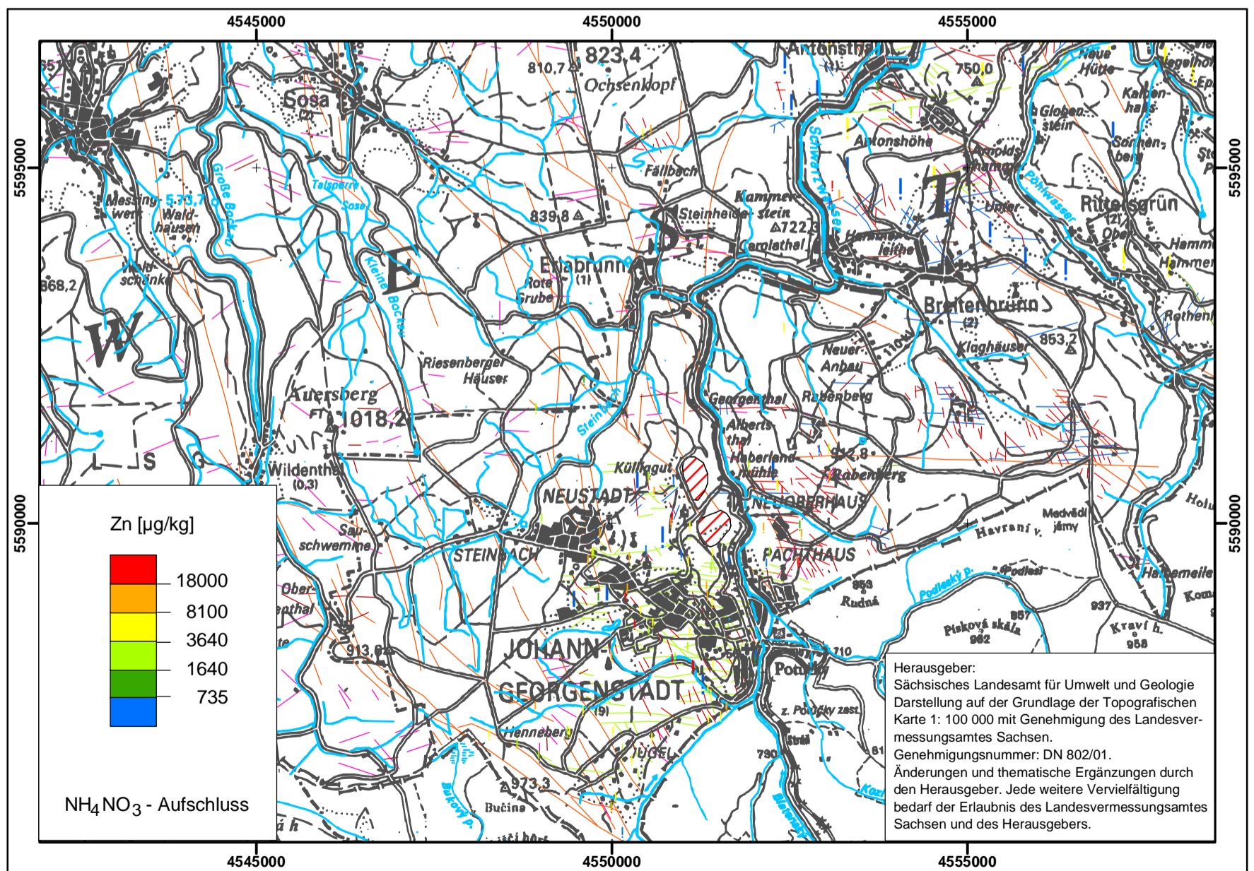
Abb. 90: Zink in den Halden
