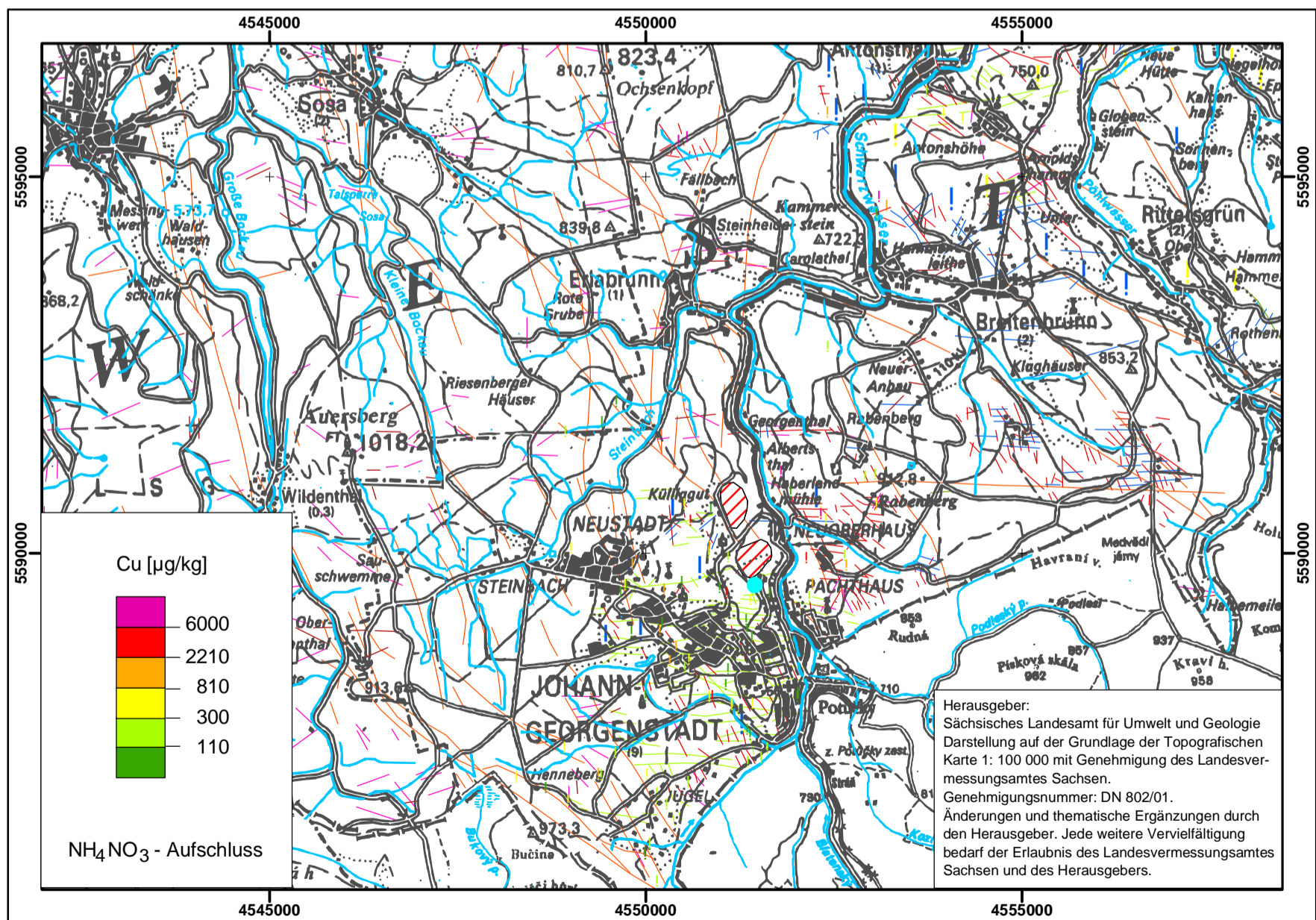
Abb. 67: Kupfer in den Halden
