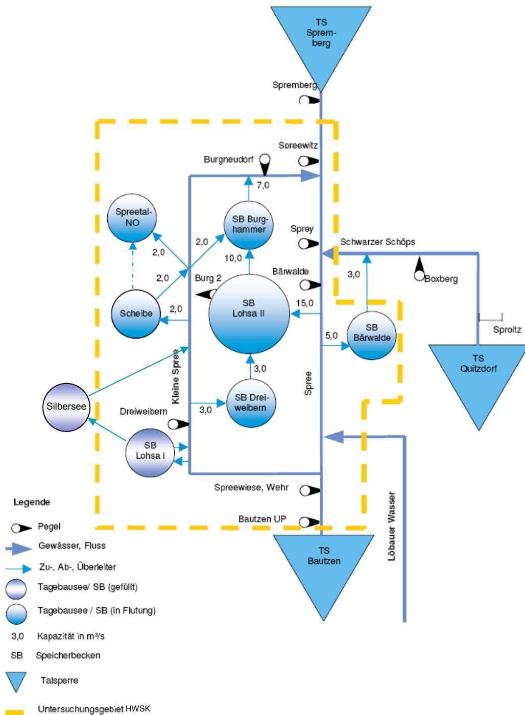
Abbildung 13: Übersicht zu Speichern und Tagebaurestseen im System Spree/ Kleine Spree (aus [4])
