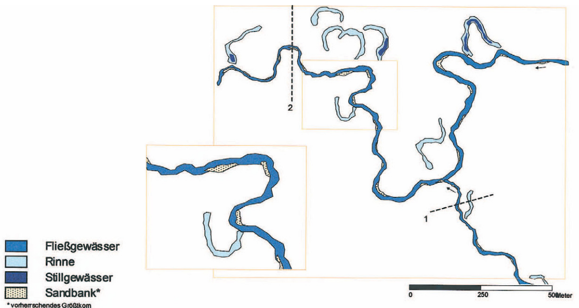
Abbildung 3: Lauform eines sandgeprägten Tieflandflusses [LUA NRW, Merkblatt 34] untersetzt mit einem Ausschnitt aus dem Kartenwerk von 1884 – Kleine Spree bei Lippitsch
